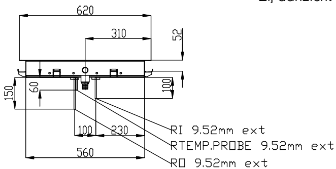
Zij aanzicht
