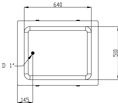
Boven aanzicht
