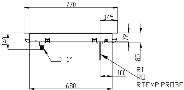
Zij aanzicht
